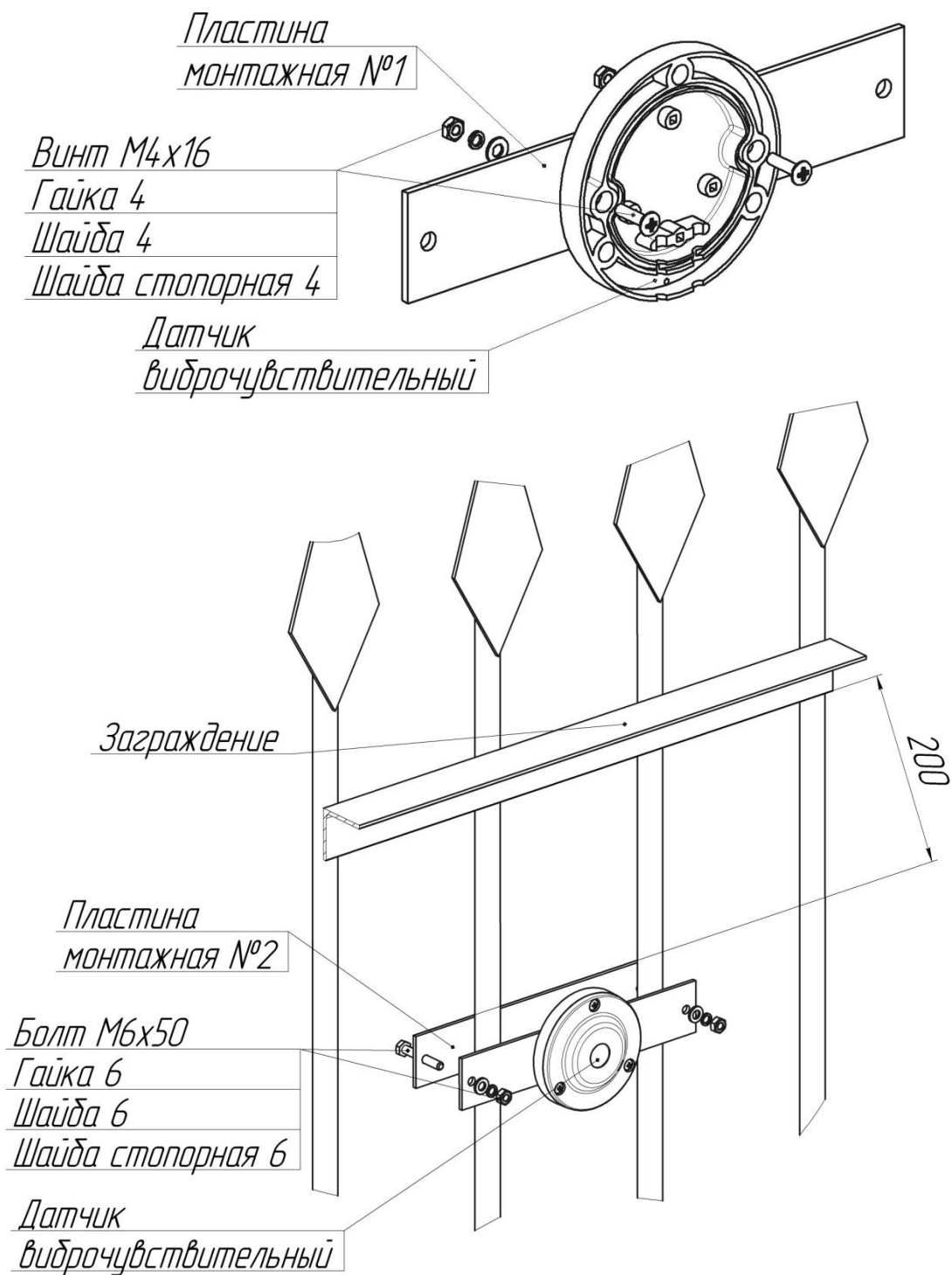
Рисунок 1 – Монтаж датчика вибросенсорного
