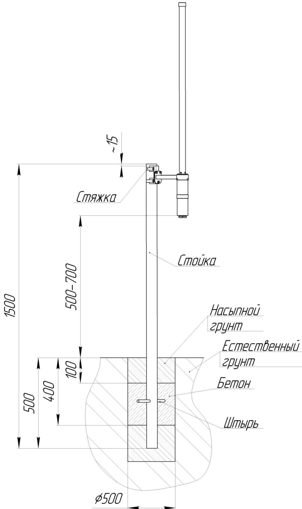
Рисунок 2 – Установка блоков извещателя
