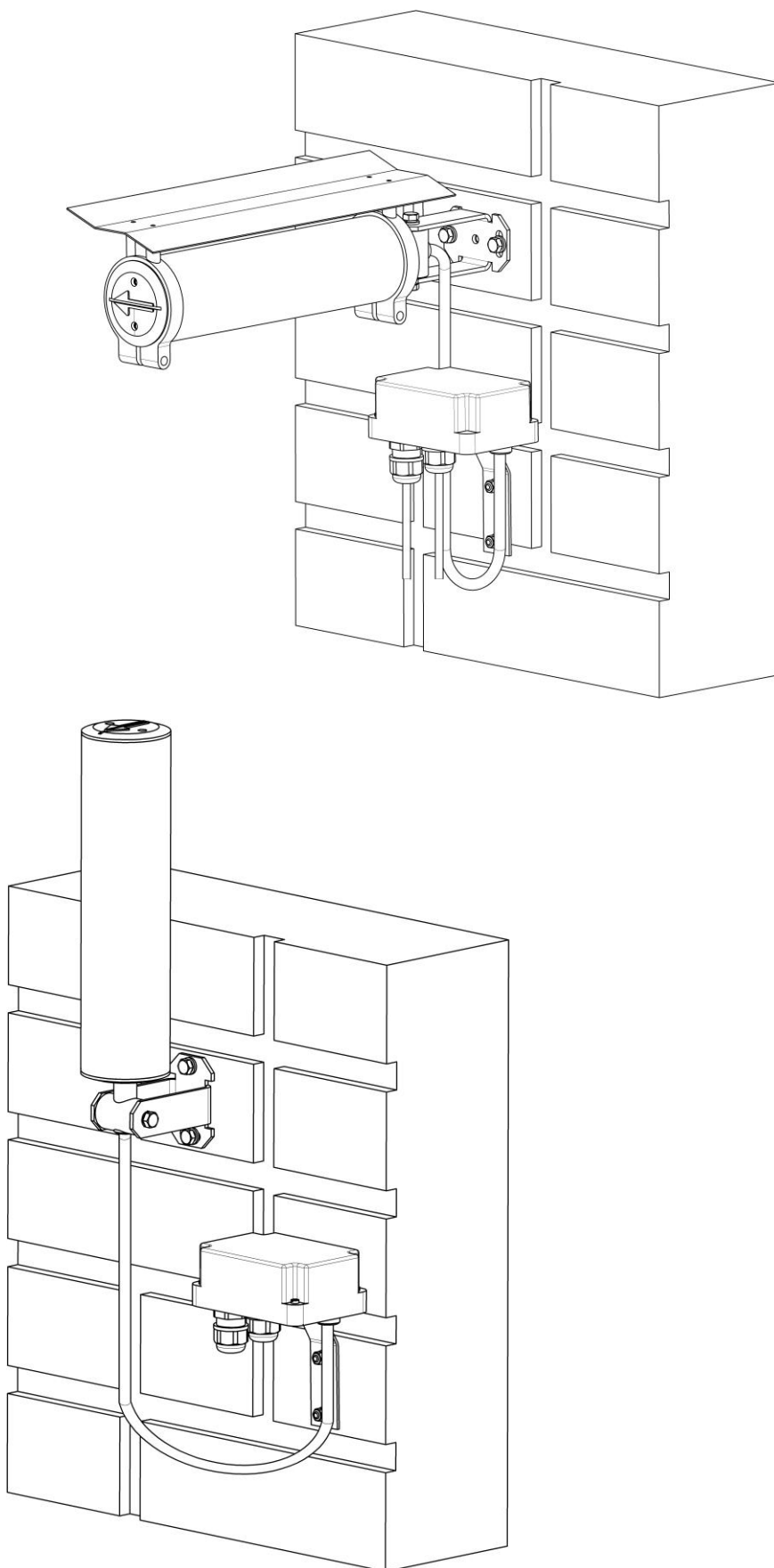
Рисунок 1.5 - Способ крепления блоков на плоской поверхности
