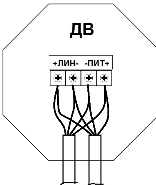
Рисунок 2.5 – Транзитное подключение ДВ
