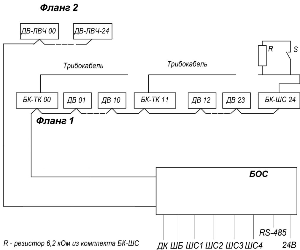
Рисунок 1.1а - Структурная схема извещателя с использованием БОС
