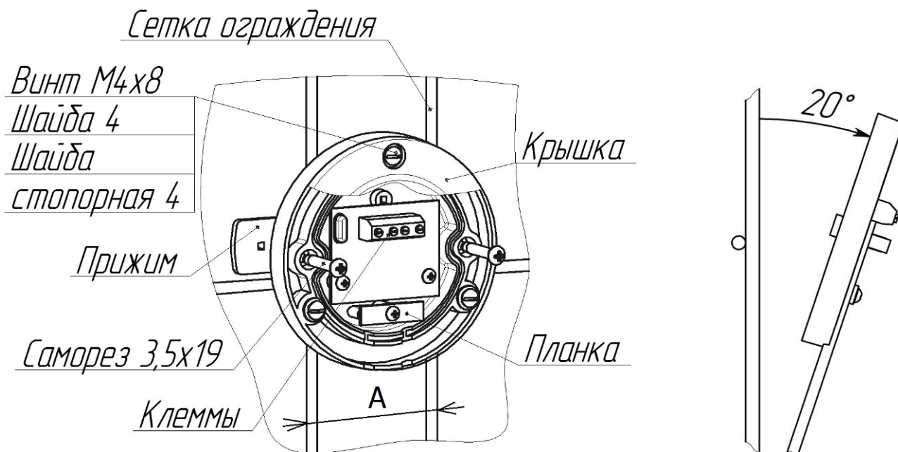
Рисунок 1.6 – Внешний вид ДВ
