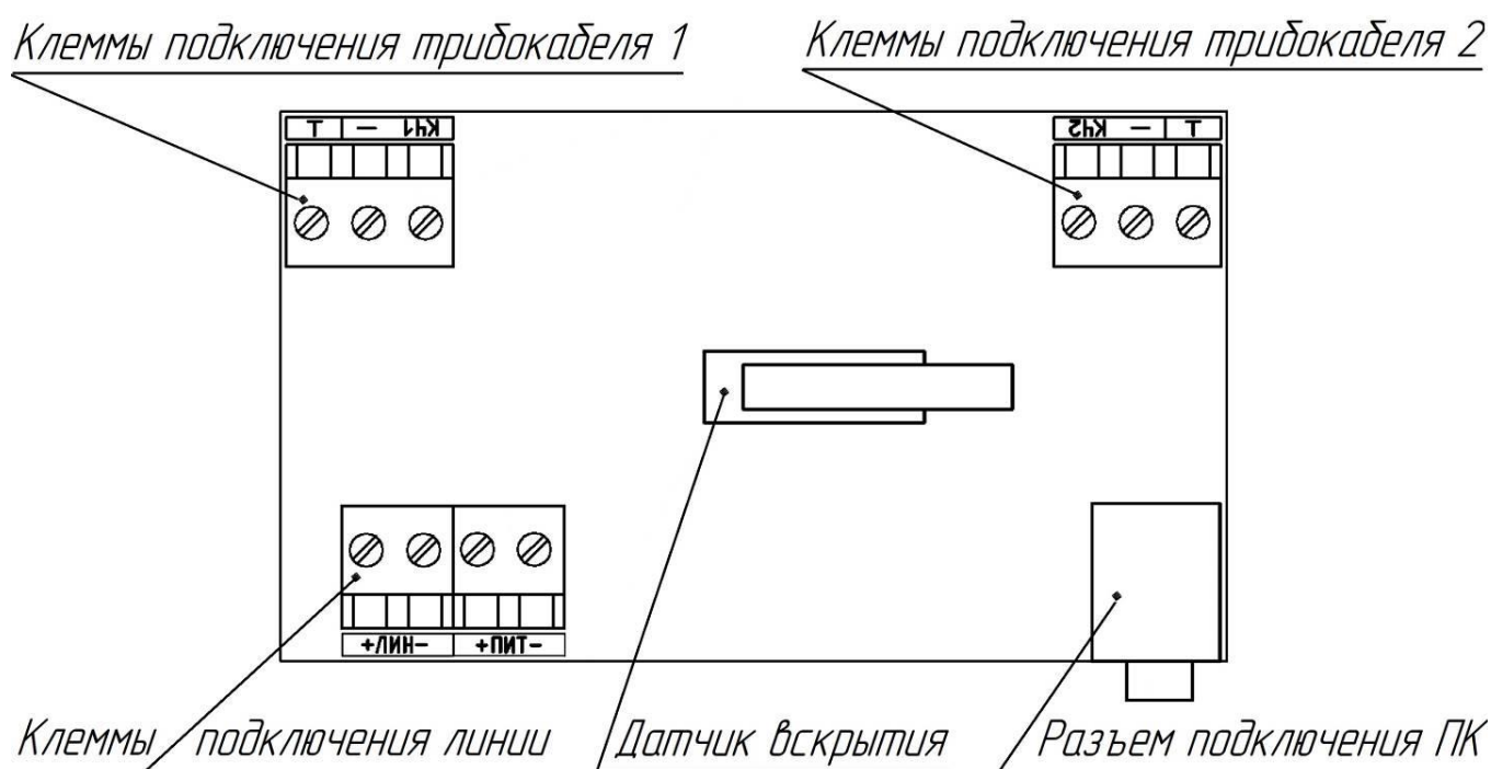
Рисунок 1.3 – Вид платы БК-ТК (БК-ТК-2)
