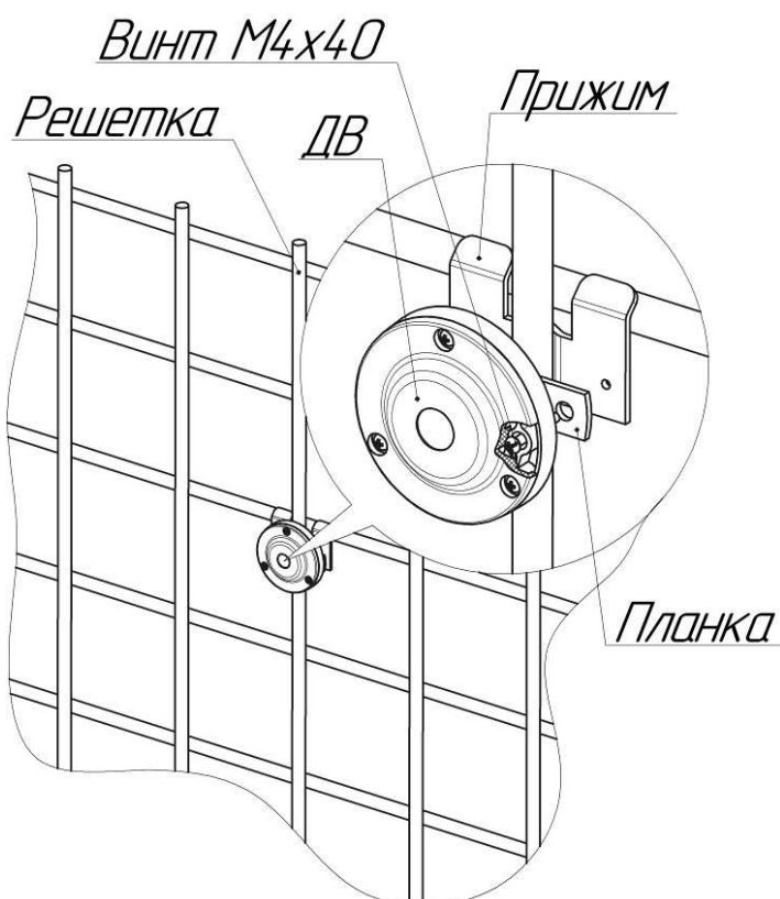
Рисунок 1.7 – ДВ на решетке
