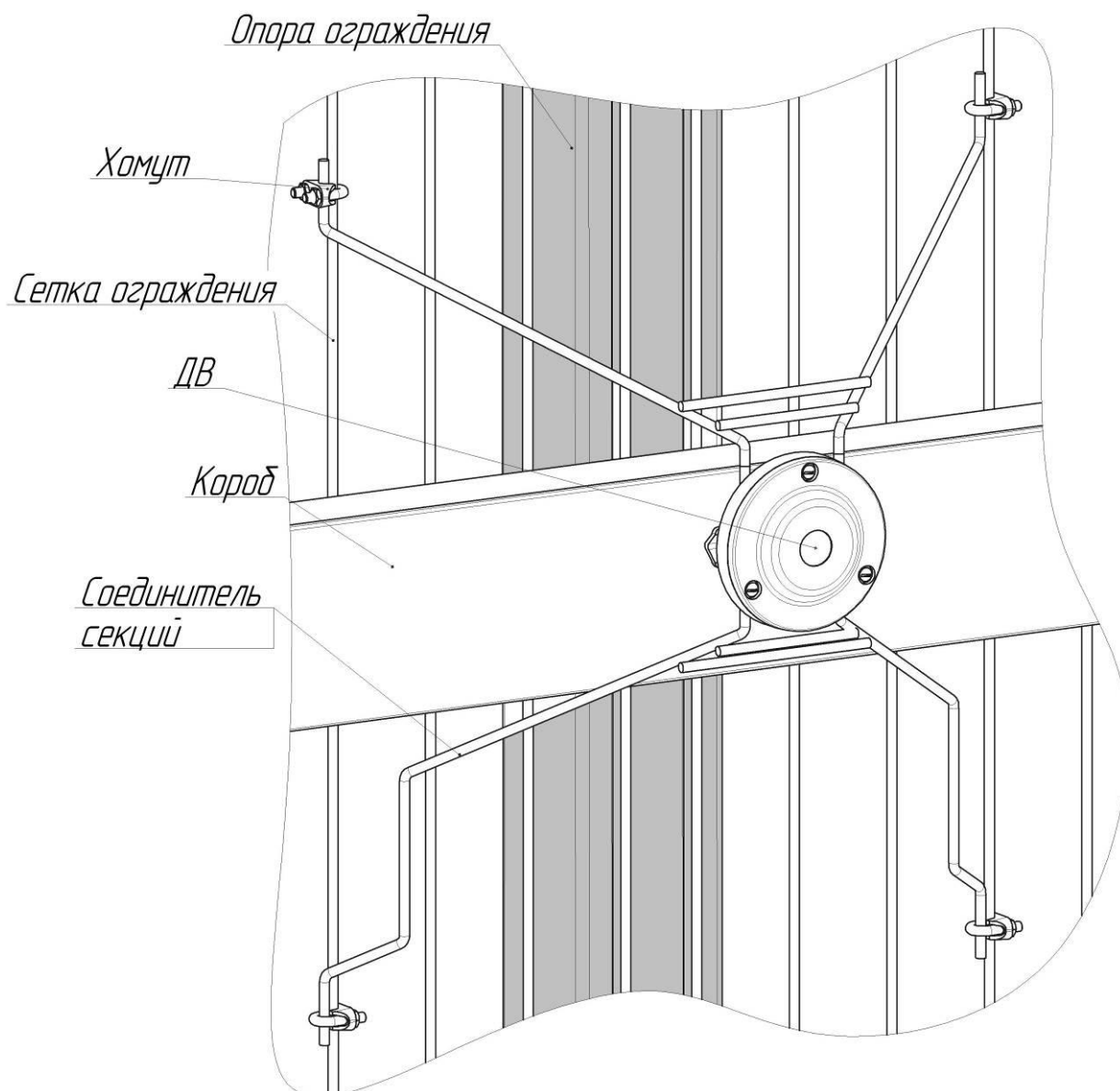
Рисунок 1.9 – Соединитель секций
