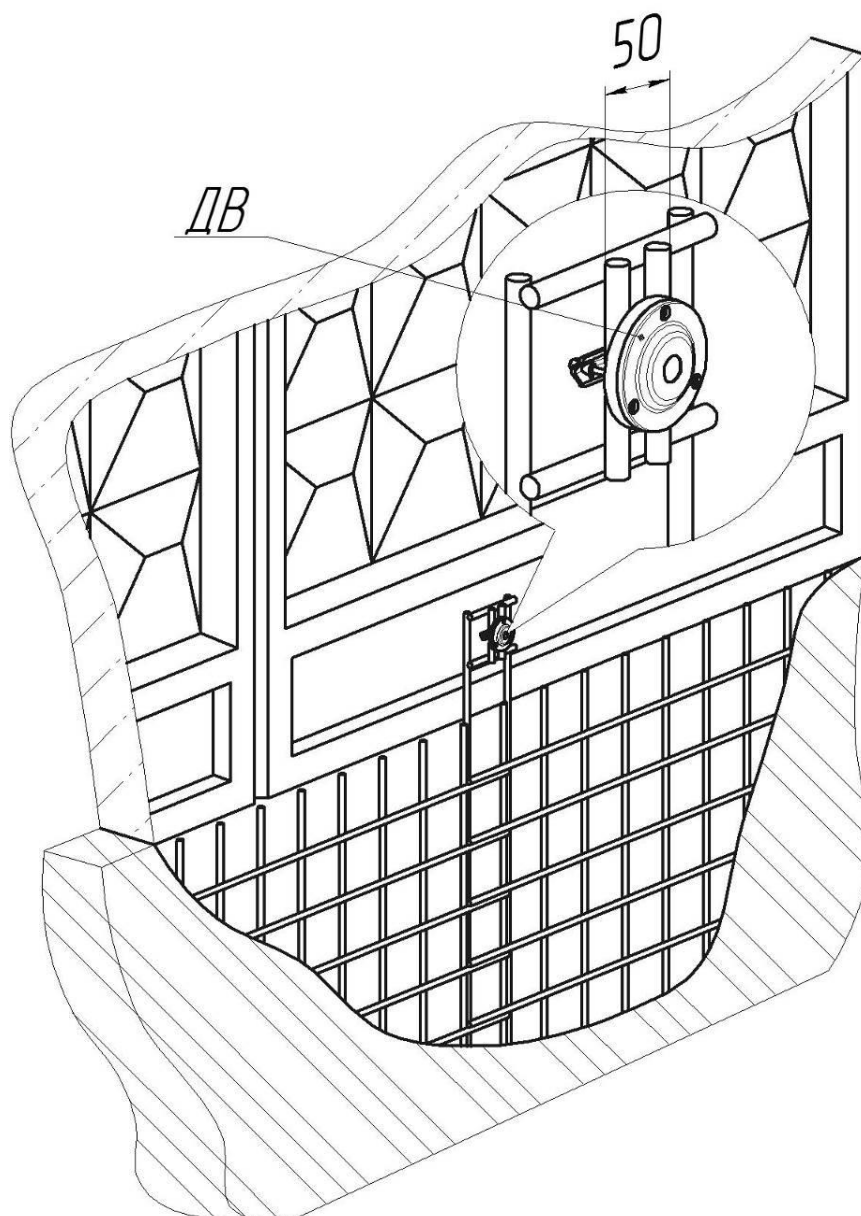
Рисунок 2.4 – Установка ДВ на решетку водопропуска
