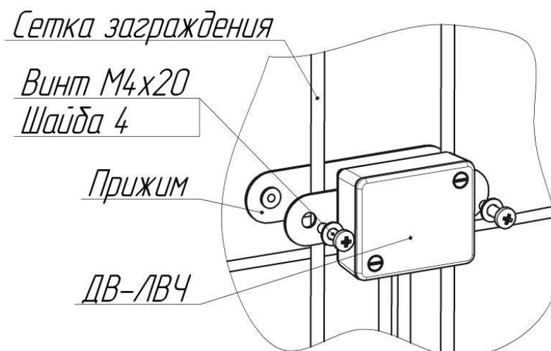
Рисунок 1.8 – Установка ДВ-ЛВЧ на заграждение
