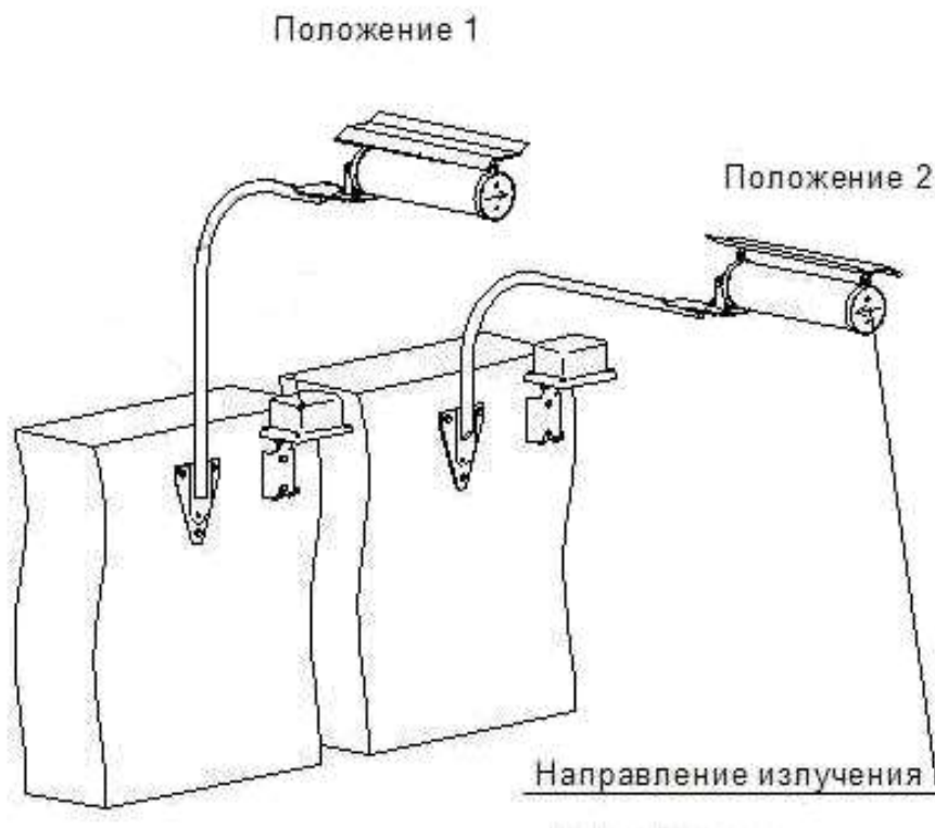
Рисунок 2.3 - Установка блоков смежных участков
