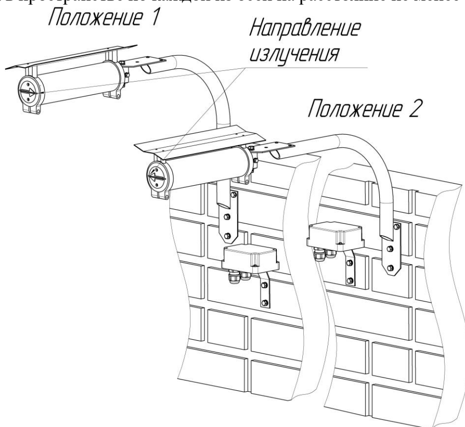
Рисунок 2.3 – Установка блоков смежных участков
