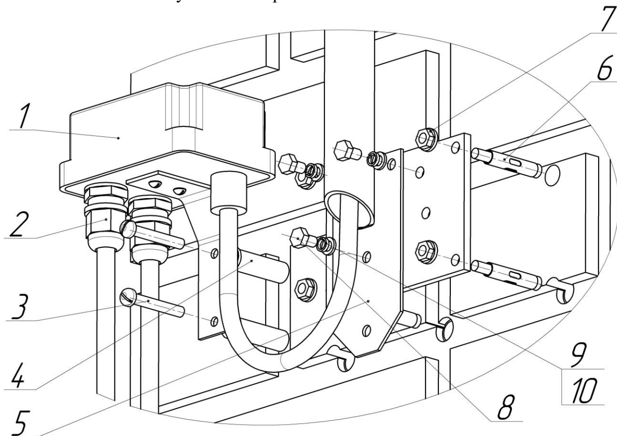
Рисунок 1.8 – Крепление блока на КМЧ-2
