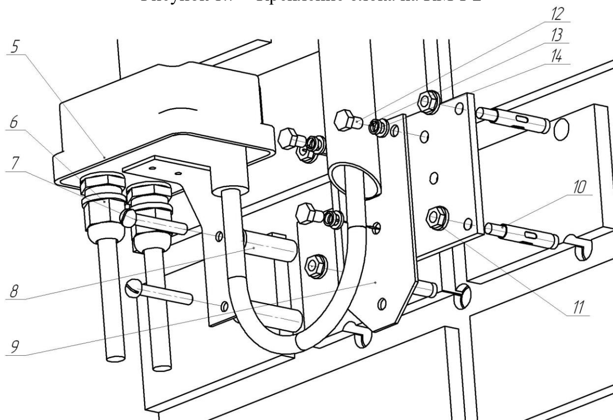
Рисунок 1.7 – Крепление блока на КМЧ-2
