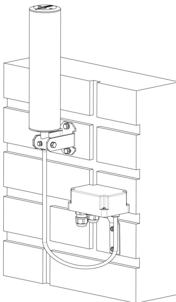
Рисунок 1.5 – Способ крепления блоков на плоской поверхности
