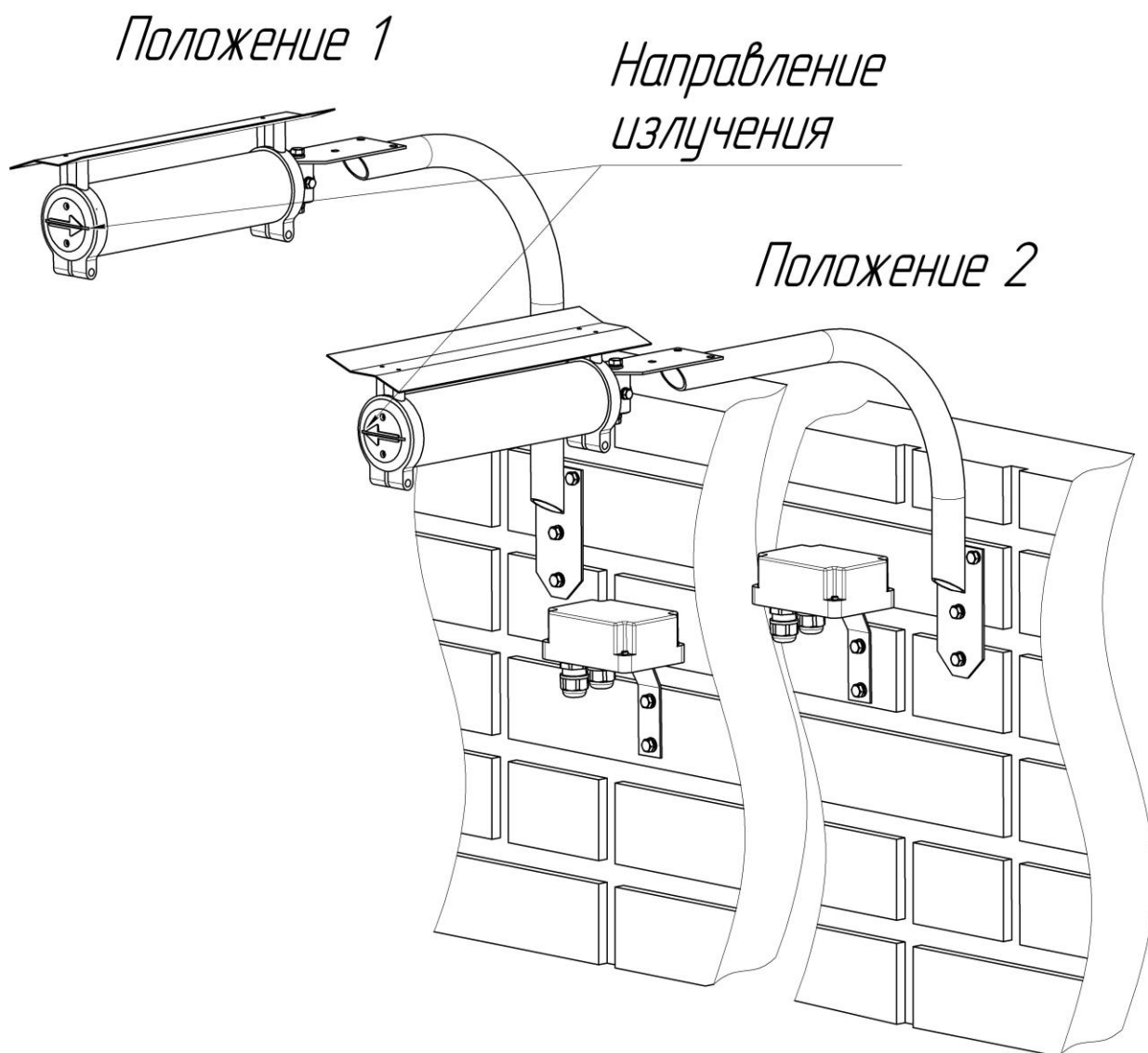
Рисунок 2.3 – Установка блоков смежных участков
