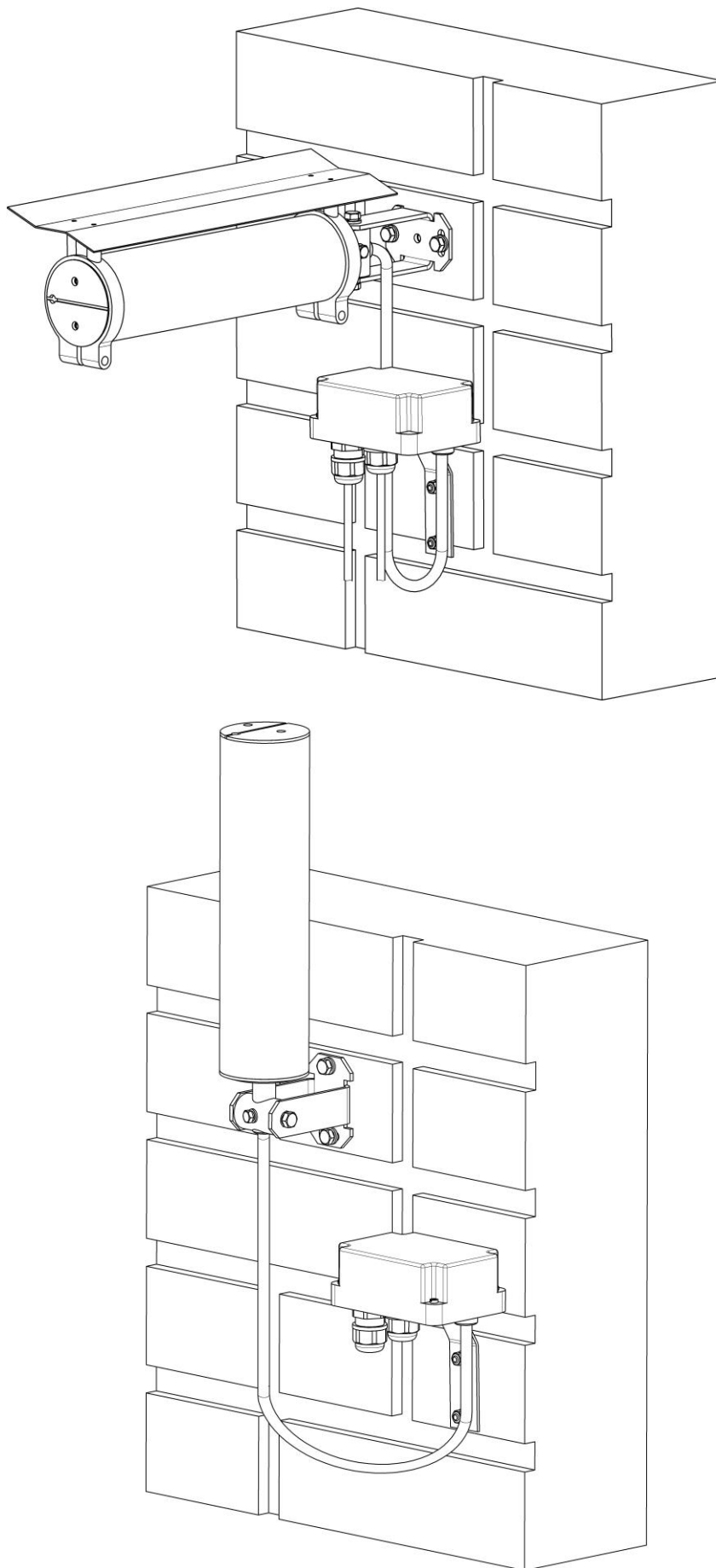
Рисунок 1.6 – Способ крепления блоков на плоской поверхности
