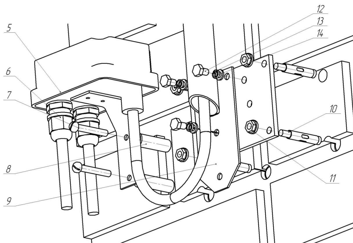
Рисунок 1.8 – Крепление блока на КМЧ-2
