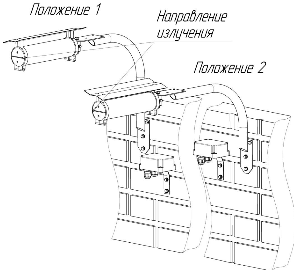
Рисунок 5.3 - Установка блоков смежных участков
