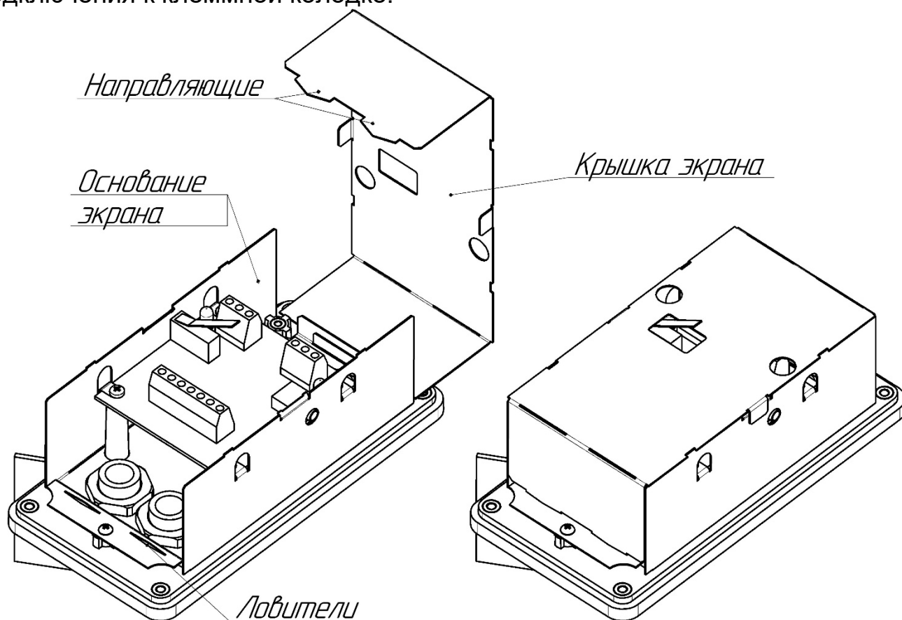
Рисунок 2.7 – Блок БК-ТК
