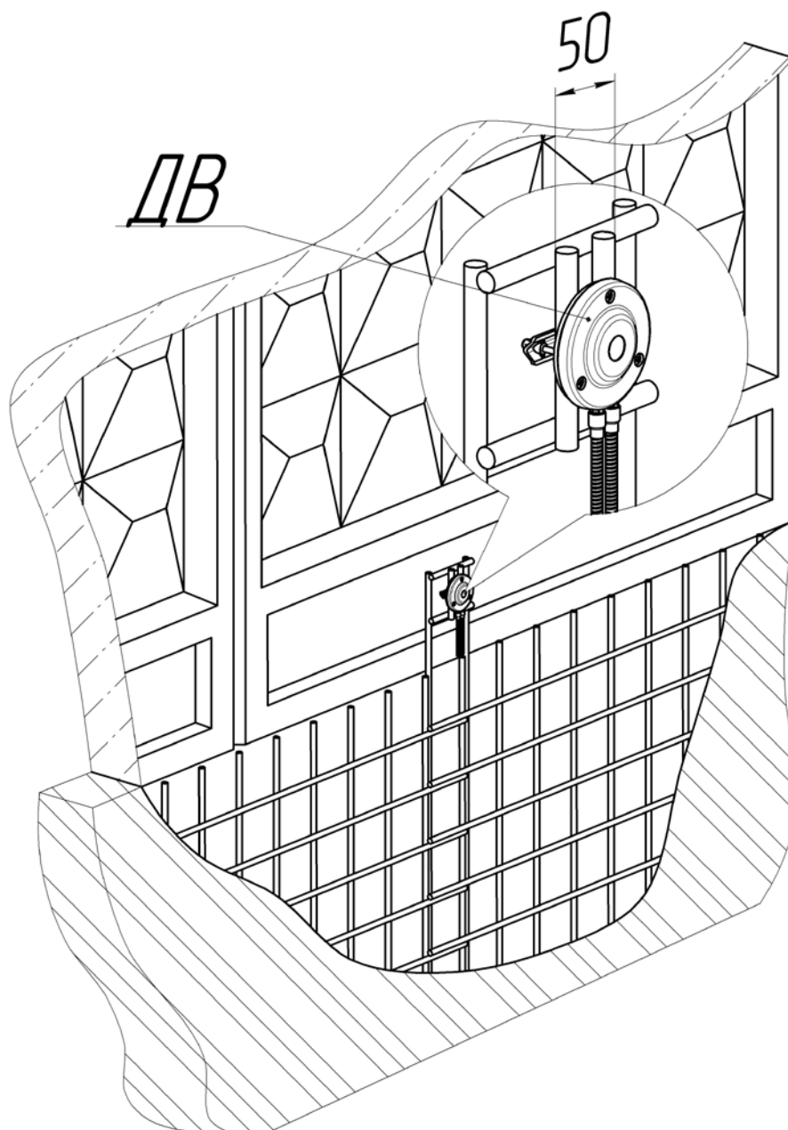
Рисунок 2.4 – Установка ДВ на решетку водопропуска
