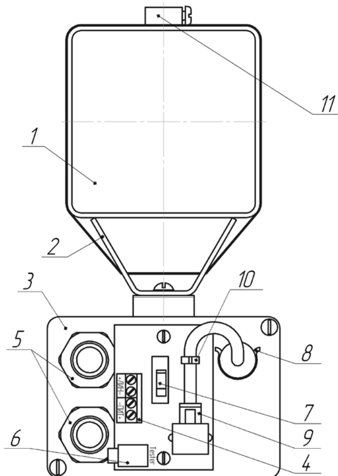
Рисунок 1.10 – Крепление БЧ на сетке
