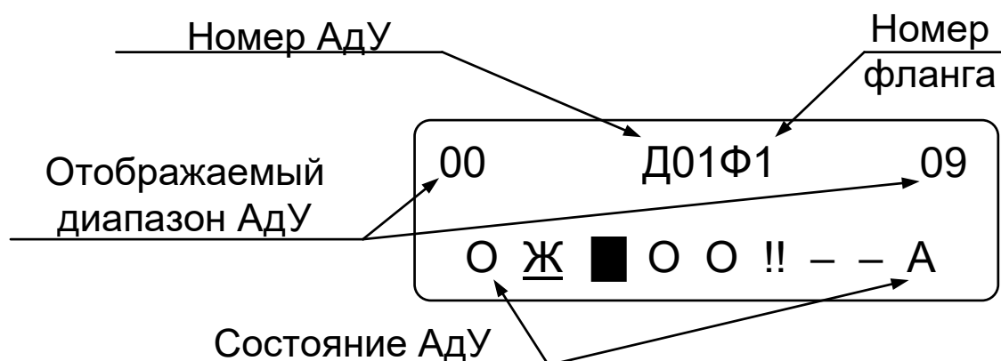
Рисунок В.2 – Окно индикации выбора АдУ
