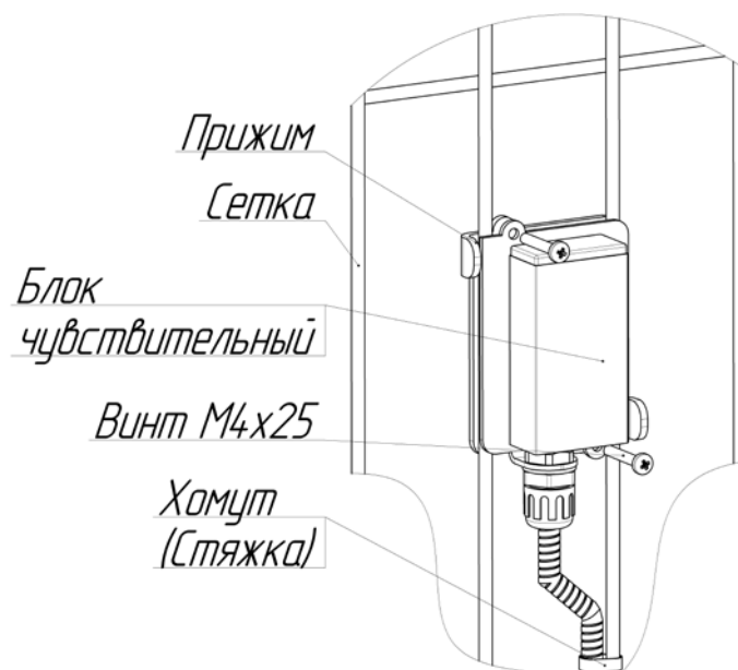
Рисунок 1.10 – Крепление БЧ на сетке
