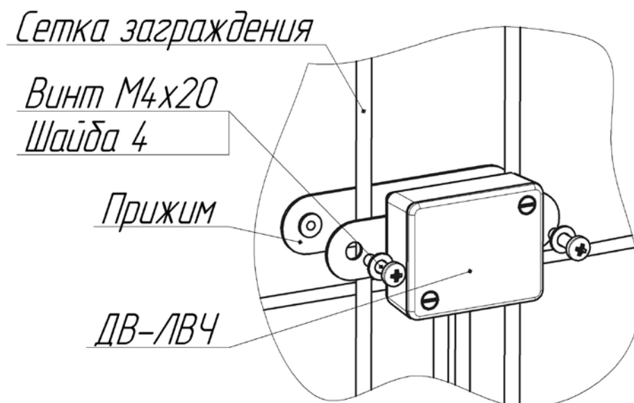
Рисунок 1.8 – Установка ДВ-ЛВЧ на заграждение
