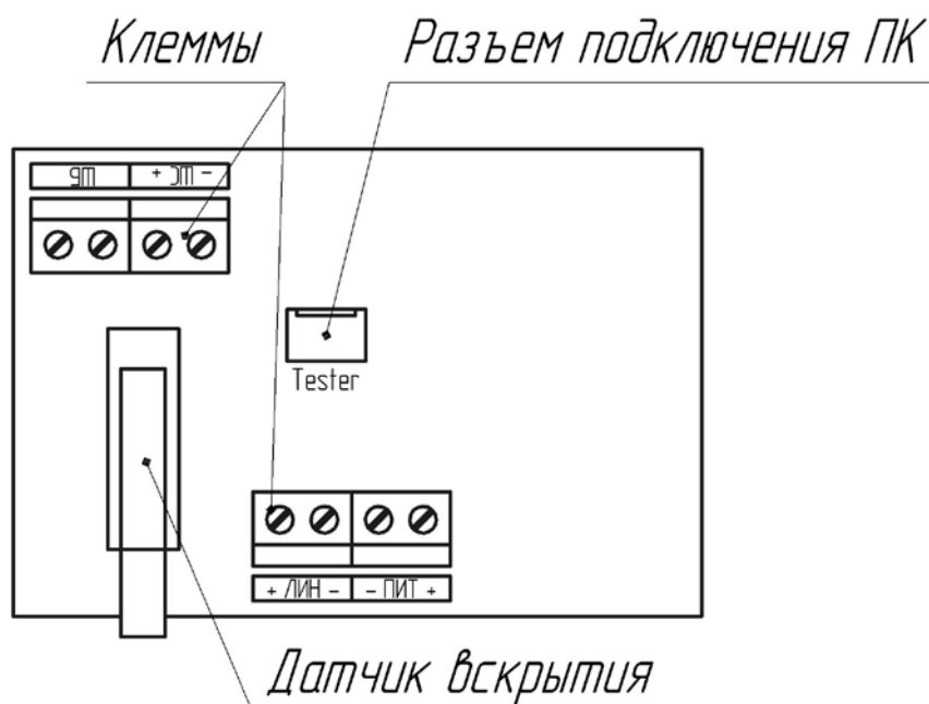
Рисунок 1.4 – Вид платы БК-ШС
