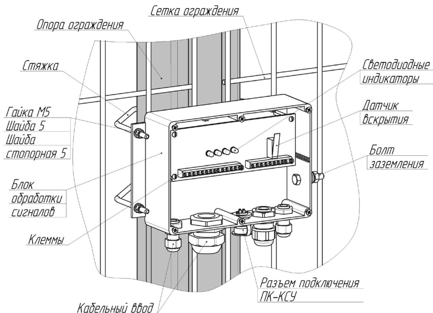
Рисунок 1.2 – Внешний вид БОС
