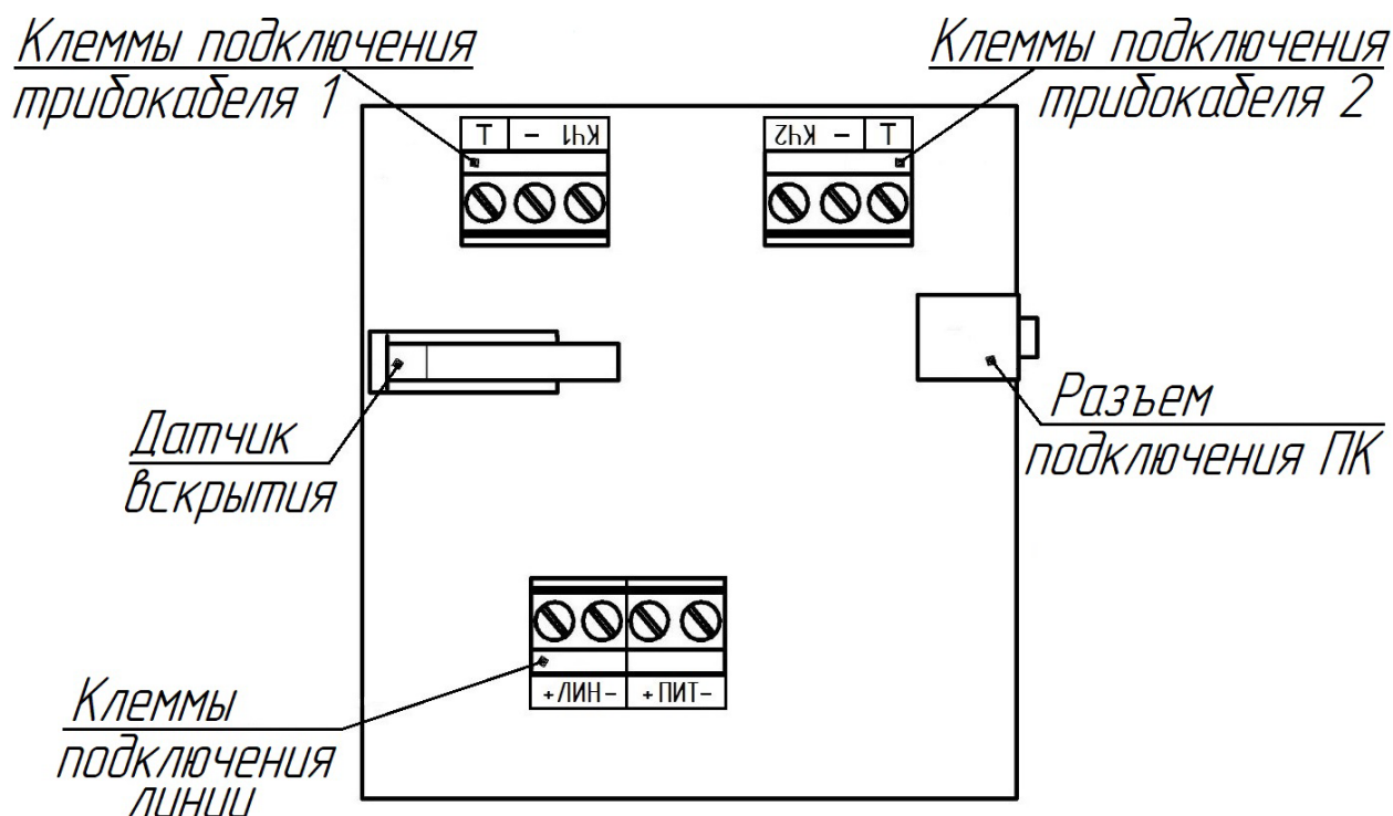
Рисунок 1.3 – Вид платы БК-ТК (БК-ТК-2)
