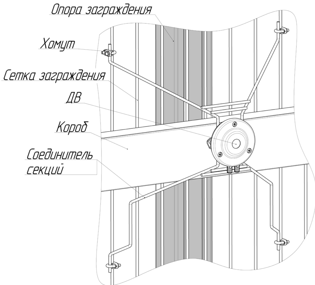
Рисунок 1.9 – Соединитель секций
