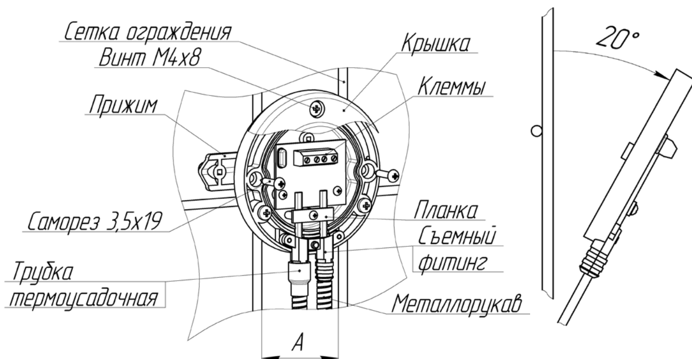
Рисунок 1.6 – Внешний вид ДВ
