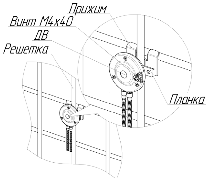
Рисунок 1.7 – ДВ на решетке
