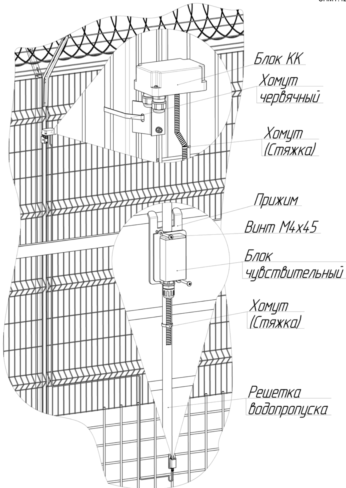
Рисунок 2.6 – Установка ДВ-Г на решетке водопропуска
