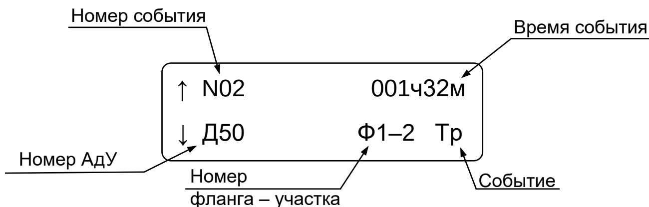
Рисунок В.4 – Окно индикации события архива
