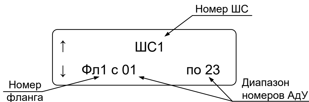
Рисунок В.5 – Окно индикации настройки работы с БР
