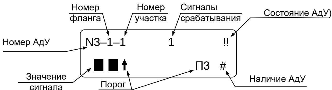
Рисунок В.3 – Окно индикации состояния и параметров АдУ
