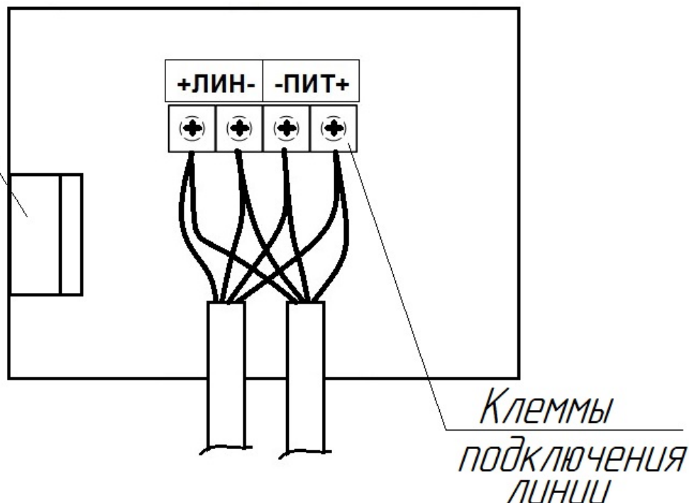
Рисунок 2.5 – Транзитное подключение ДВ
