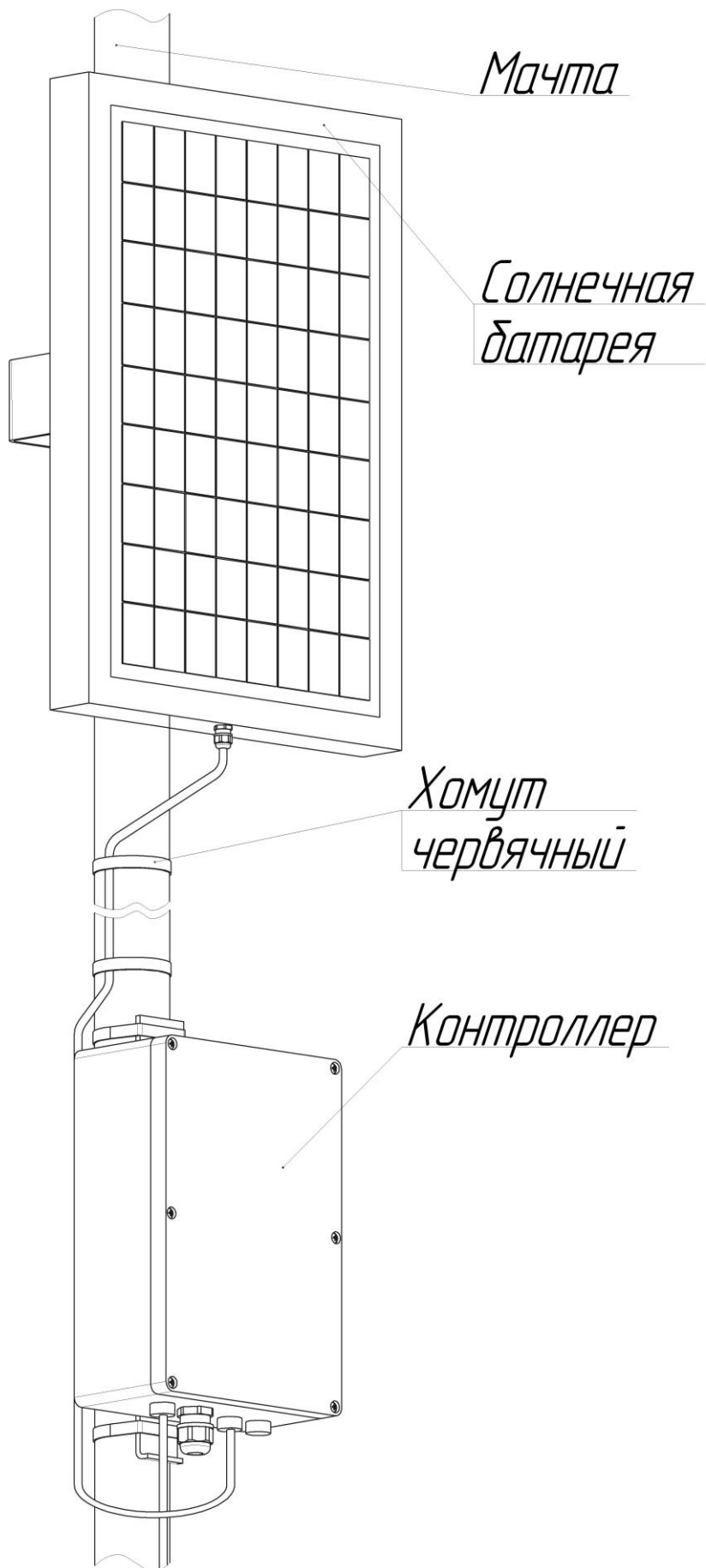
Рисунок 1 – Крепление БАП-С на мачте (опоре)
