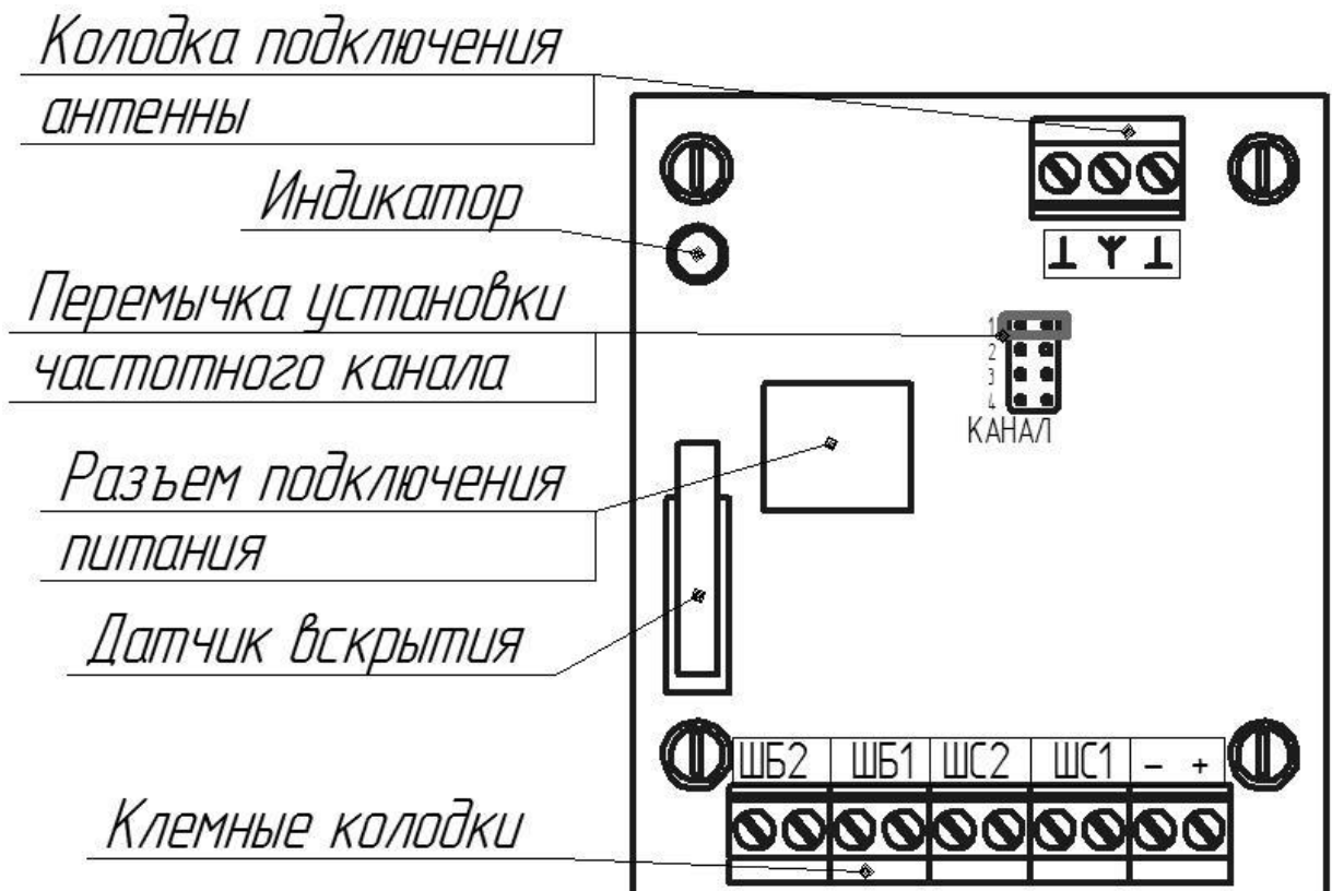
Рисунок 2 – Панель РМ-ПРМ
