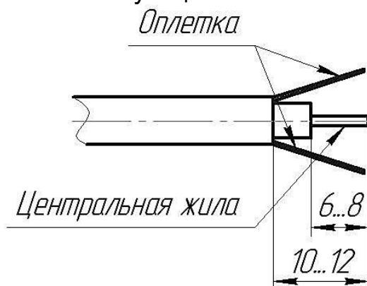
Рисунок 3 – Разделка антенного кабеля
