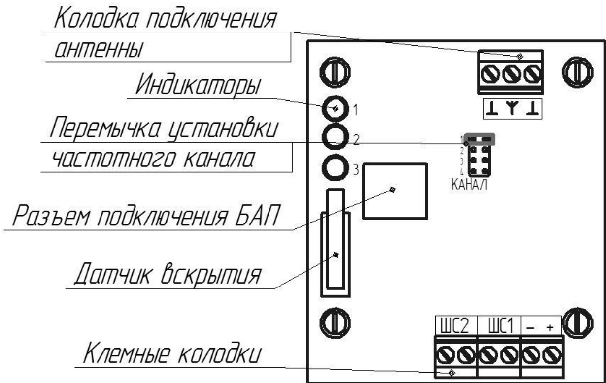
Рисунок 1 – Панель РМ-ПРД
