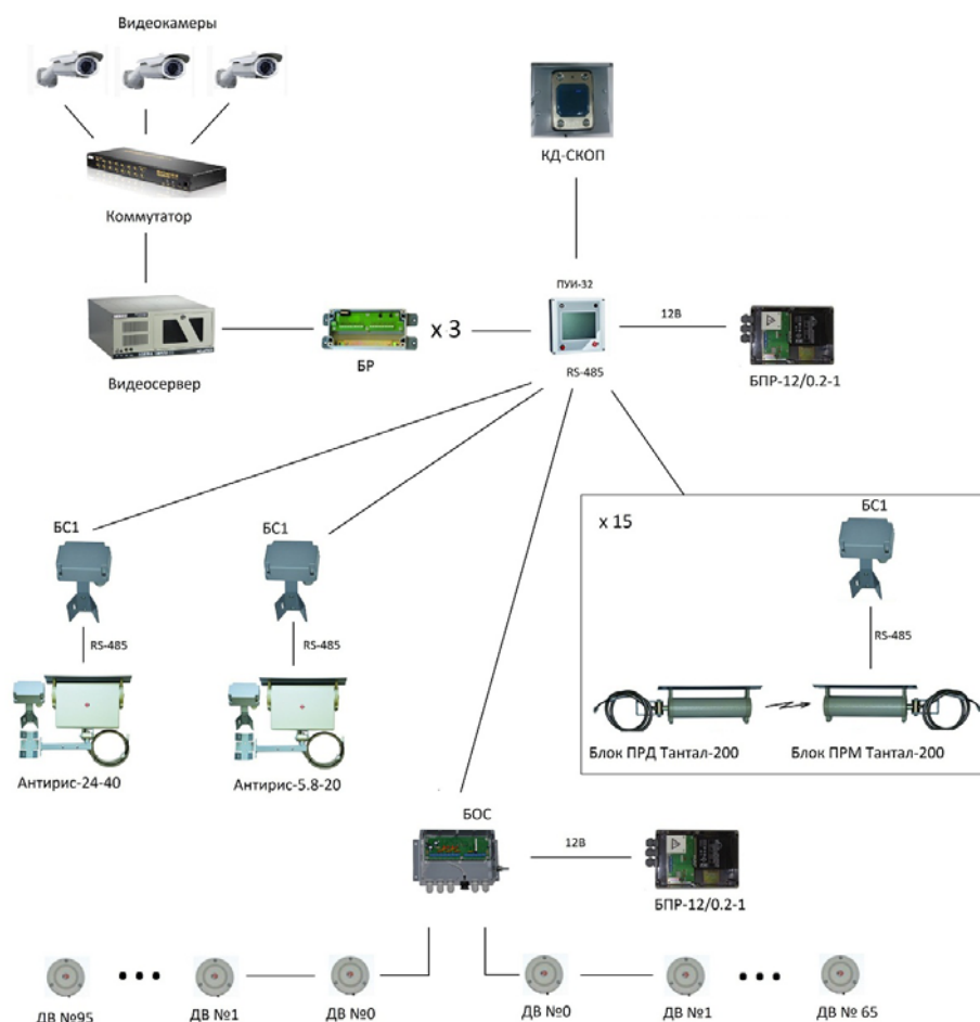
Рисунок 12– Структурная схема охранного оборудования основного участка периметра
