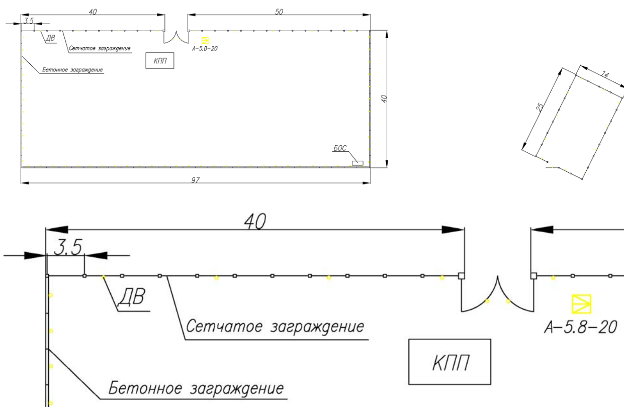
Рисунок 7 – Схема оснащения объекта охранными извещателями
