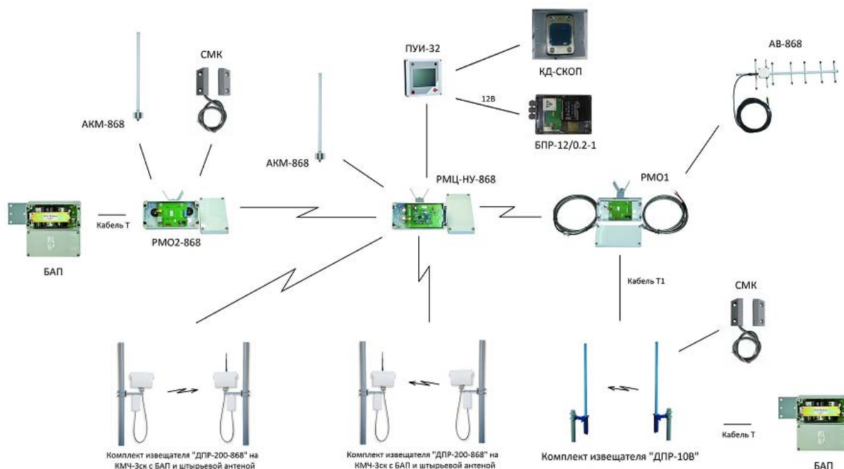
Рисунок 6 – Структурная схема охранного оборудования
