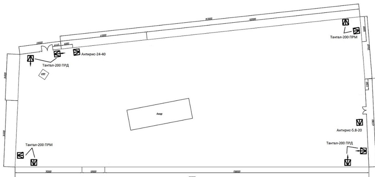
Рисунок 2 – Схема оснащения объекта охранными извещателями
