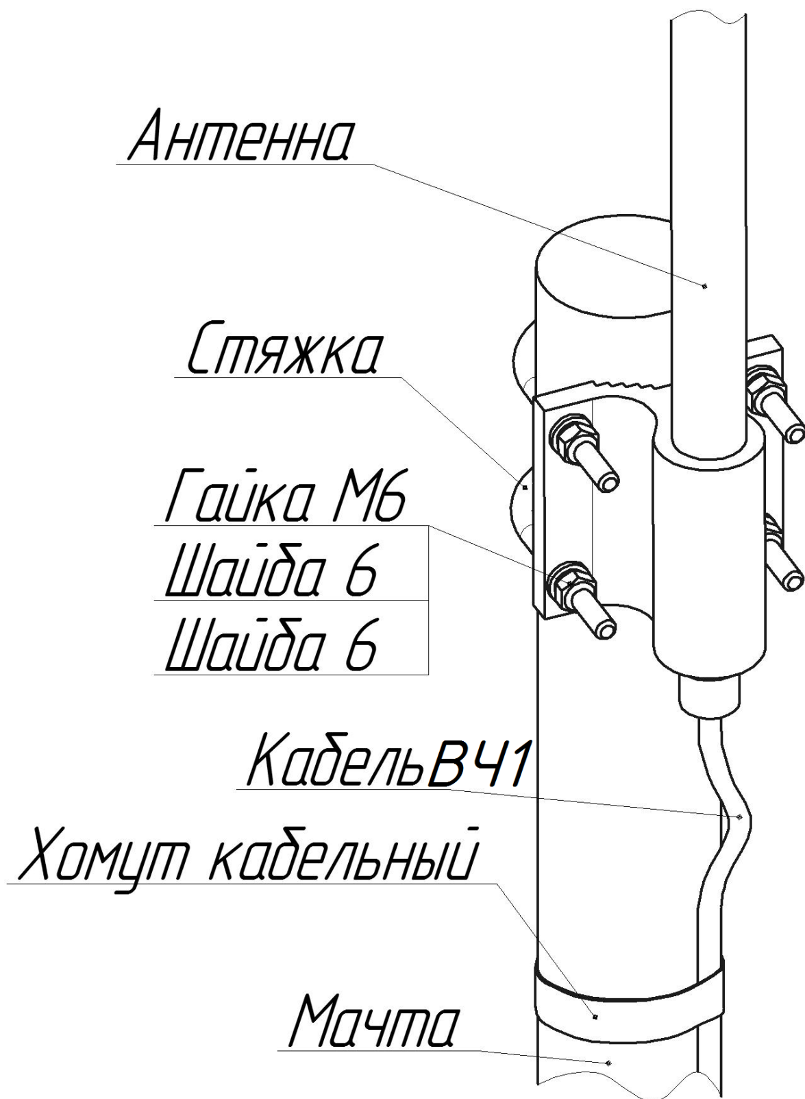
Рисунок 1 – Установка Комплекта Антенны АКМ-433 на мачте
