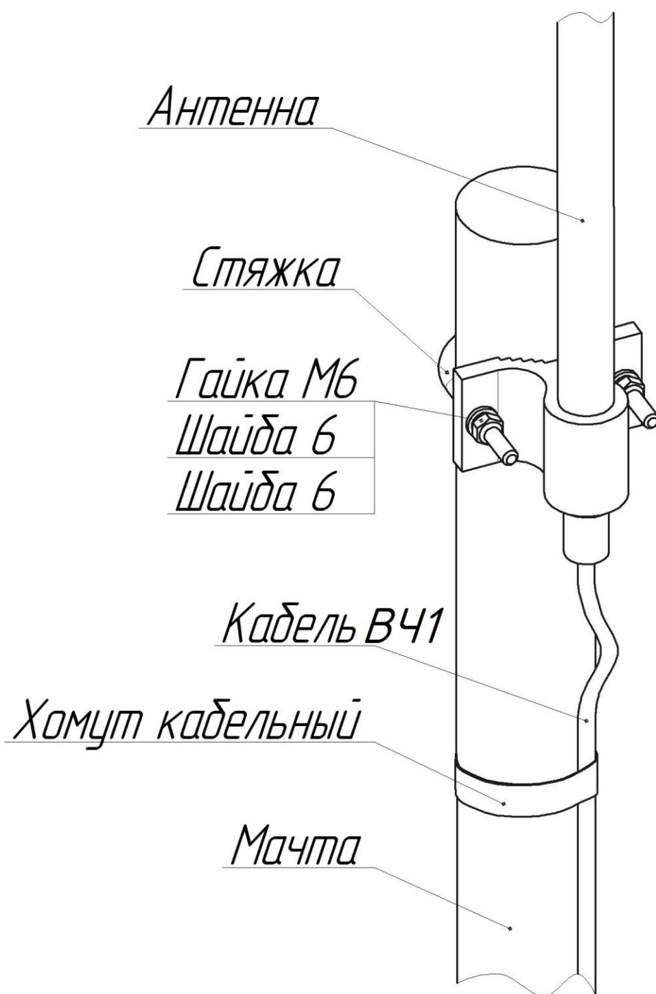
Рисунок 1 – Установка Комплекта Антенны АКМ-868 на мачте
