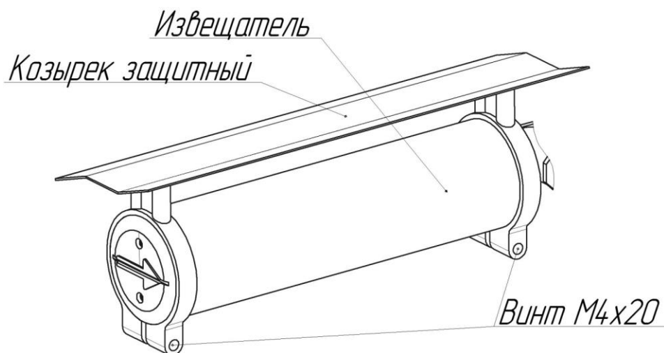
Рисунок 1- Вид блока извещателя с защитным козырьком
