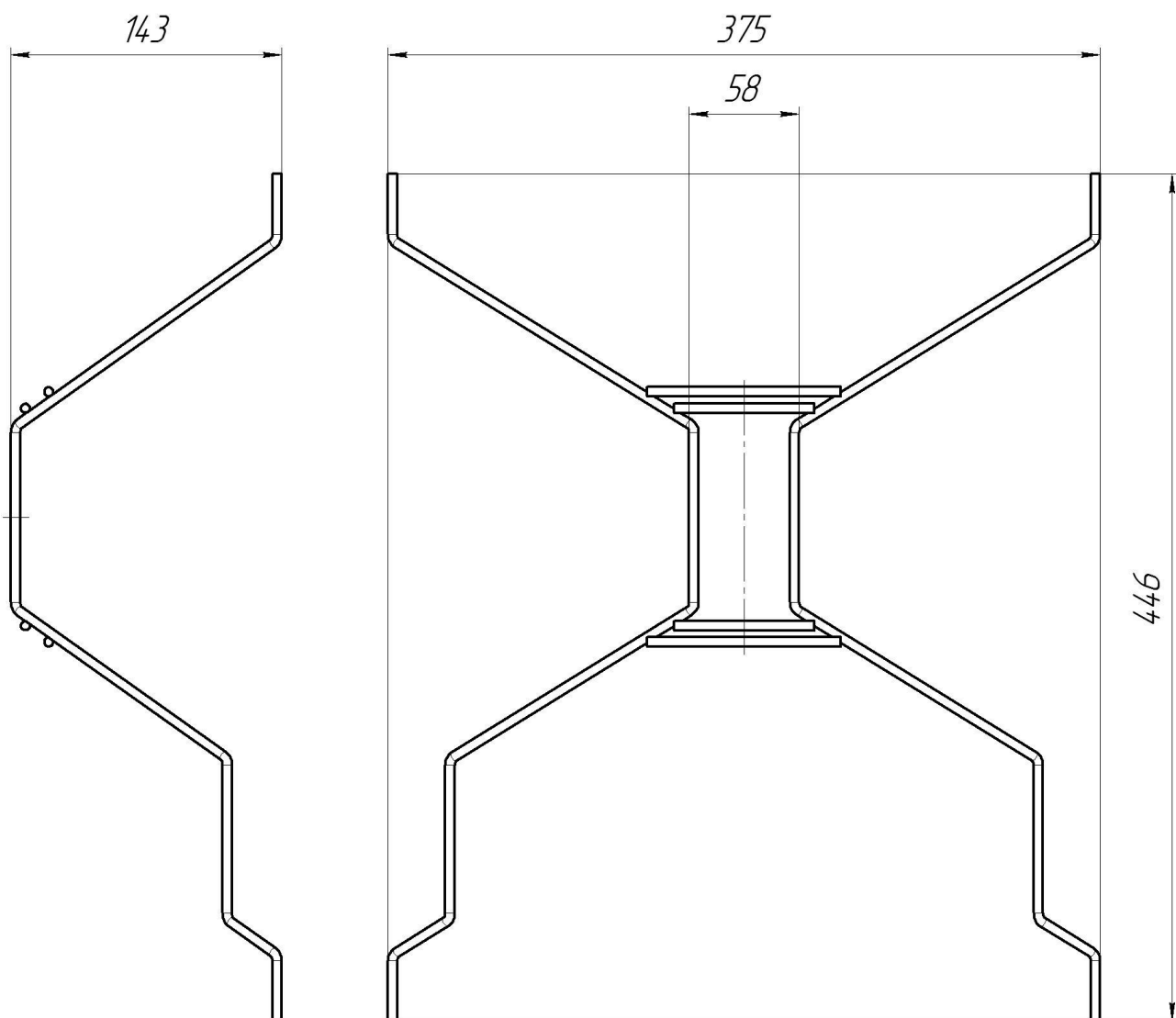
Рисунок 1 – Соединитель секций
