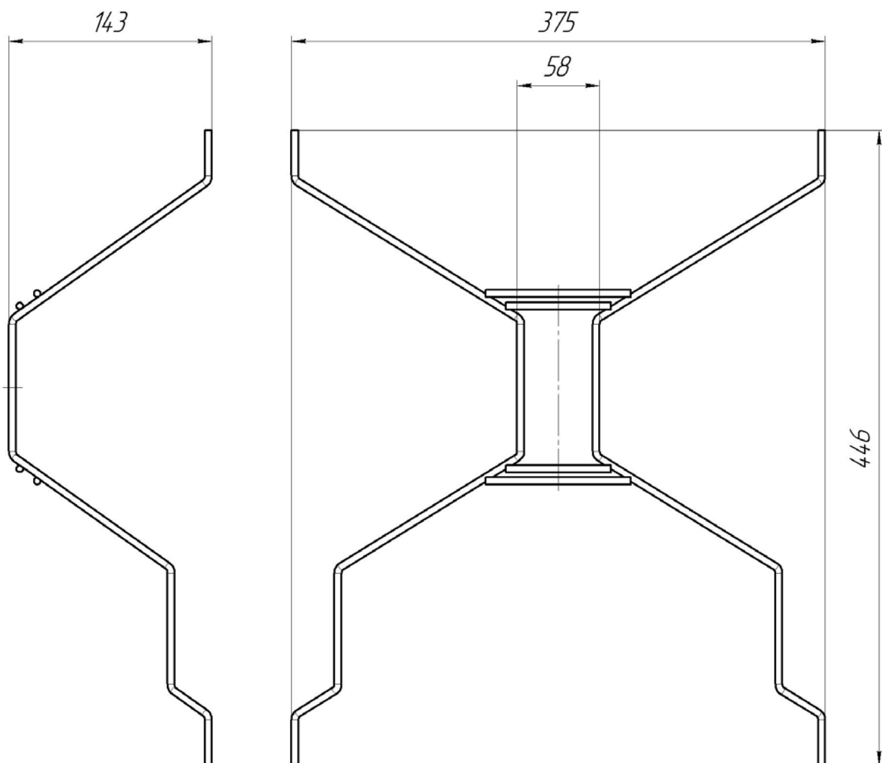
Рисунок 1 – Соединитель секций
