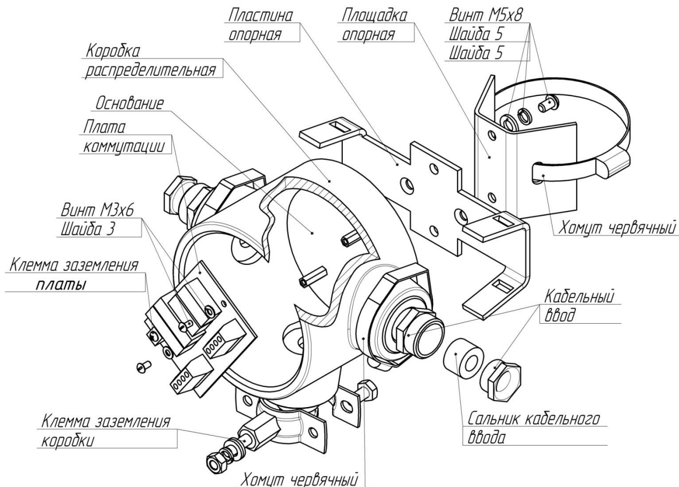
Рисунок 1– Комплект взрывозащиты
