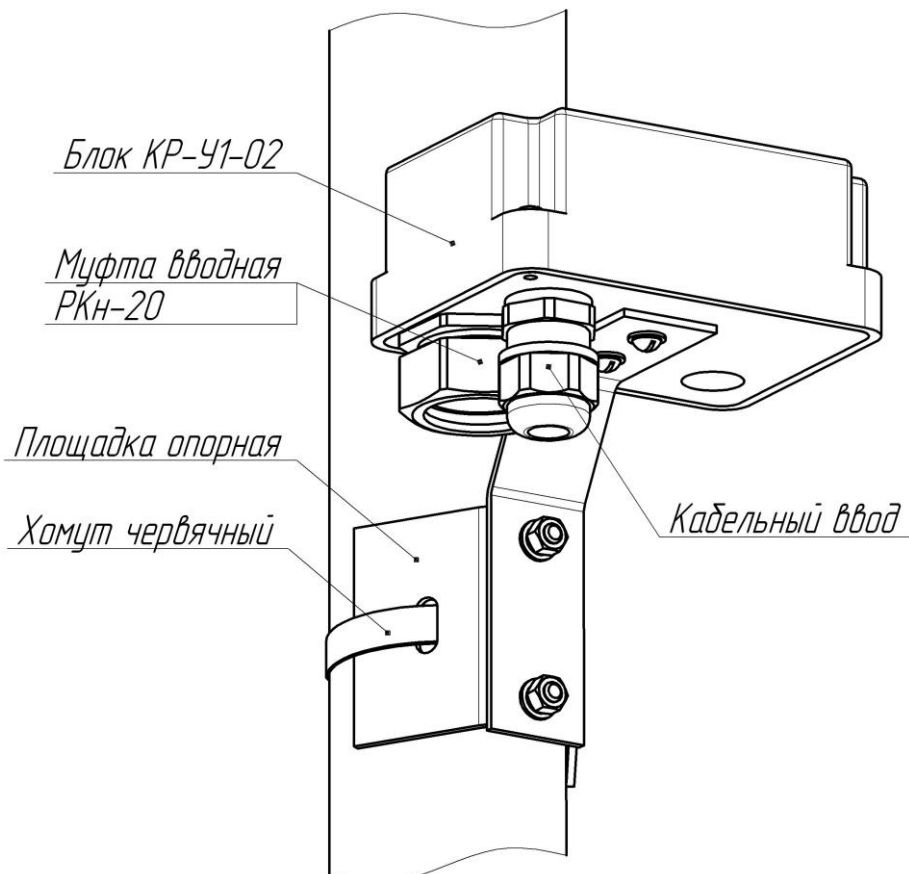
Рисунок 1 – Установка КР-У1-02 на круглой опоре
