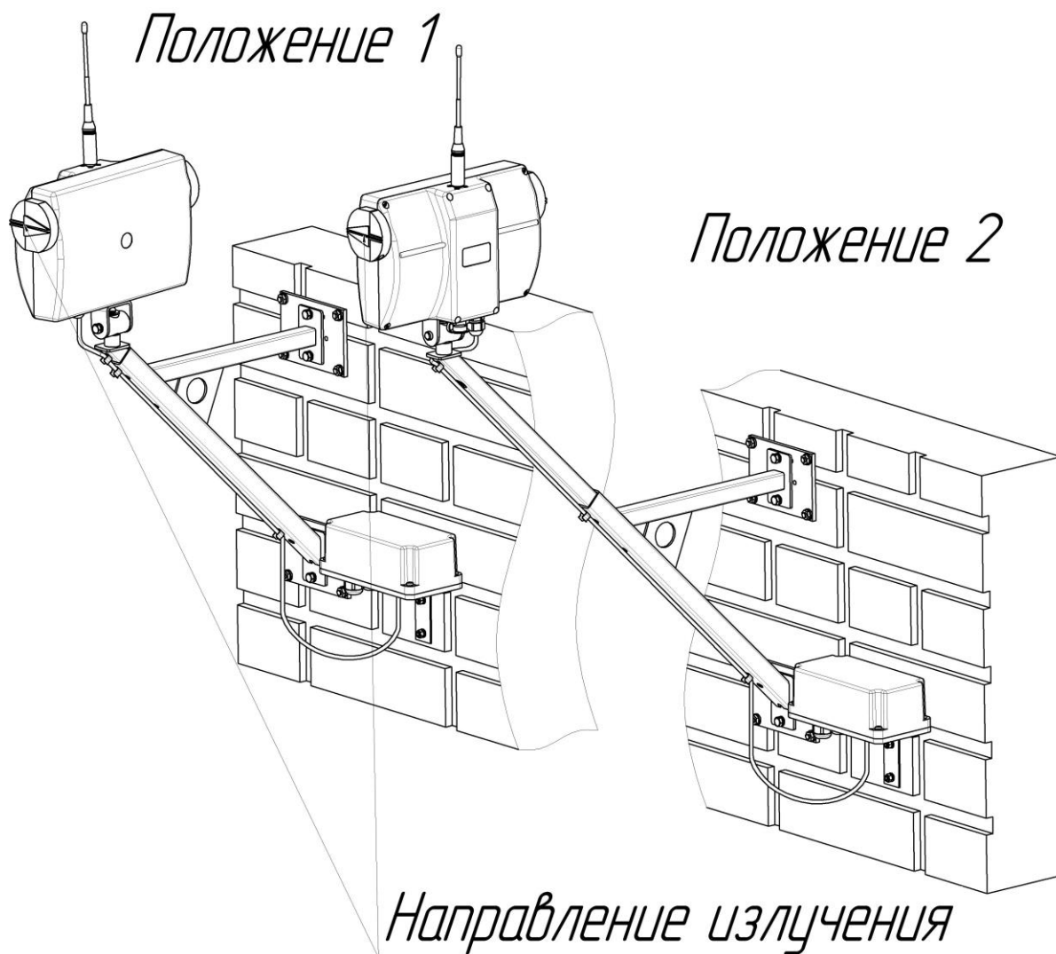
Рисунок 2.3 - Установка блоков смежных участков
