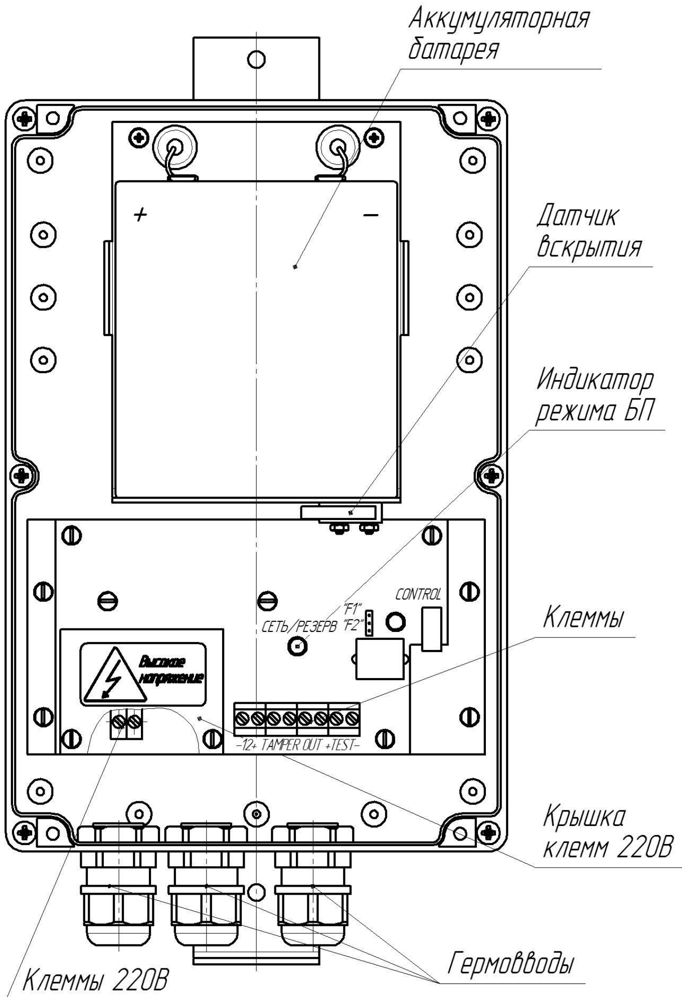
Рисунок 1 – Вид БП со снятой крышкой
