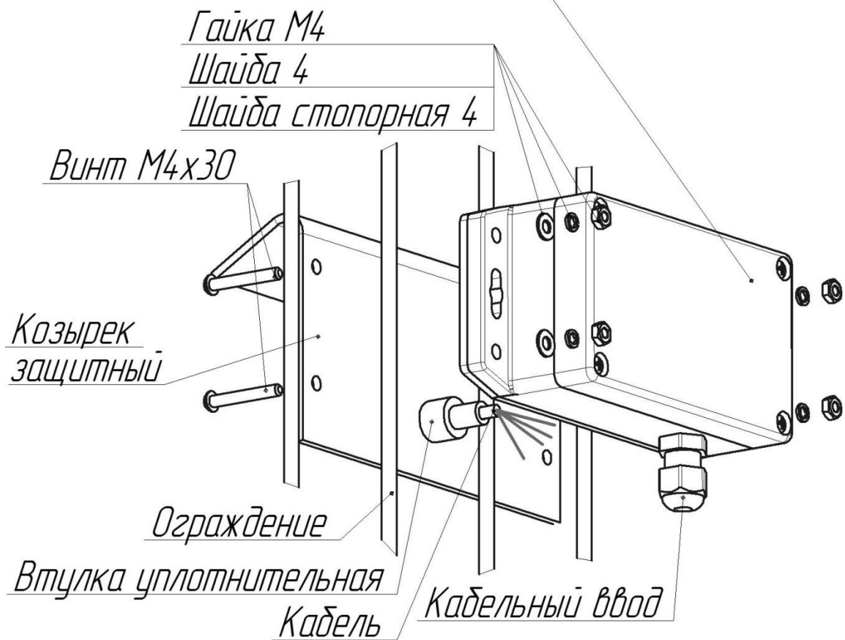
Рисунок 2 – Крепление считывателя
