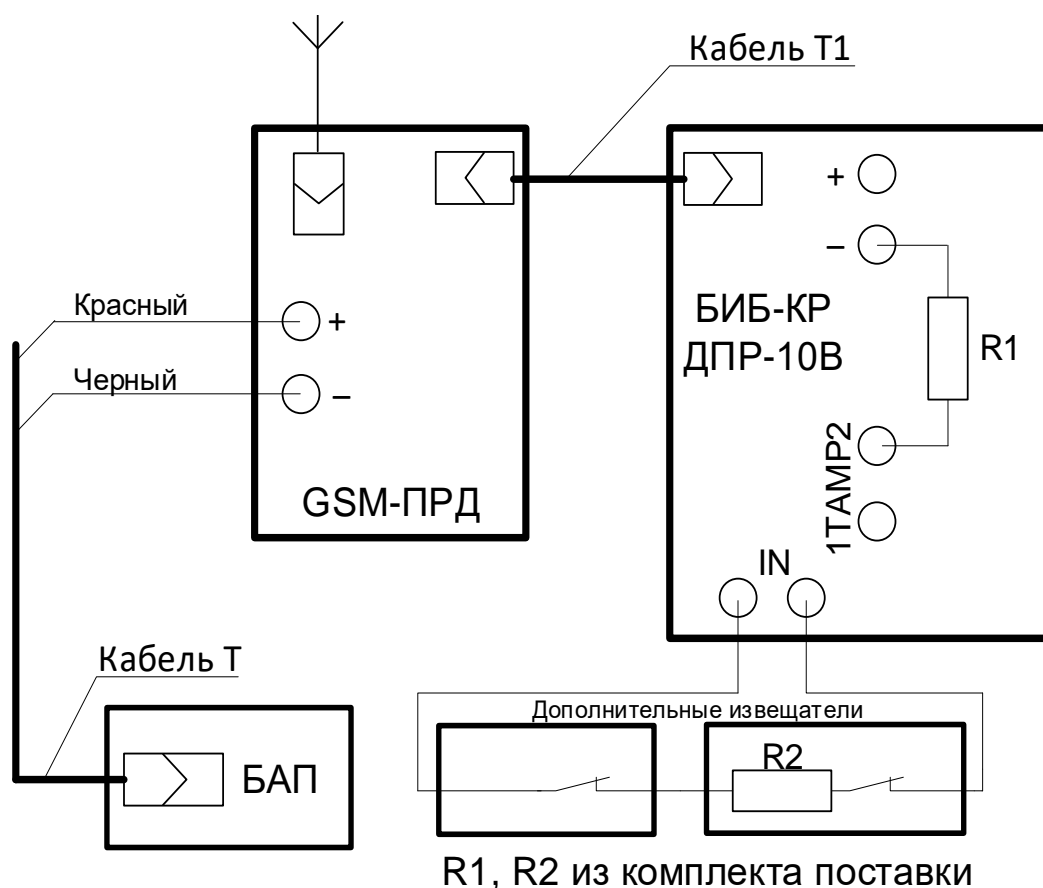
Рисунок 4 – Подключение ДПР-10В
